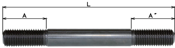
(寸法表)
