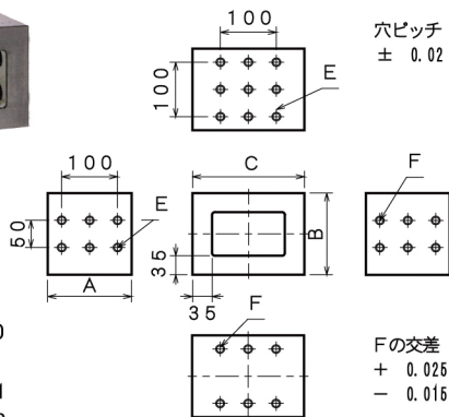
(寸法表)
