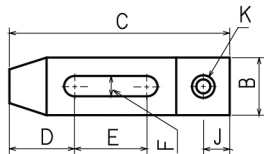
(寸法表)
